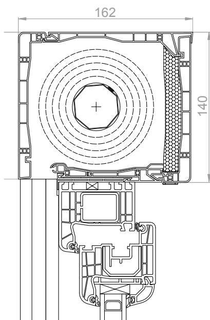
VÝŠKA SCHRÁNKY 140 MM
